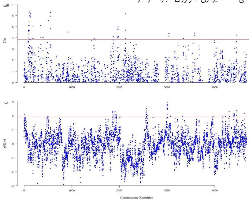
شکل ۱- نمودار منهن پلات نواحی ژنومی شناسایی شده به عنوان نشانههای انتخاب در کروموزوم X در شتر تک کوهانه ایرانی با استفاده از روش ZFst (الف) و XP-EHH (ب)؛ خط قرمز نشان دهنده حد آستانه معنادار برای هر یک از روش ها است
