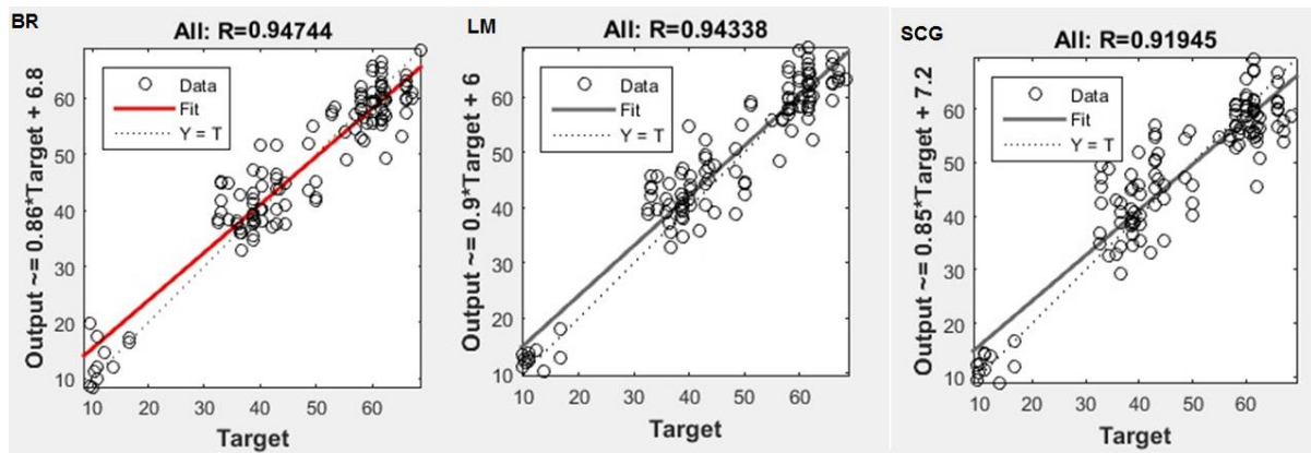
شکل ۳- دقت شبکه عصبی آموزش داده شده با الگوریتم آموزش بیزی BR، لونبرگ مارکوات LM و اسکیلد کانژوگیت گرادینت SCG (به ترتیب از چپ به راست)
