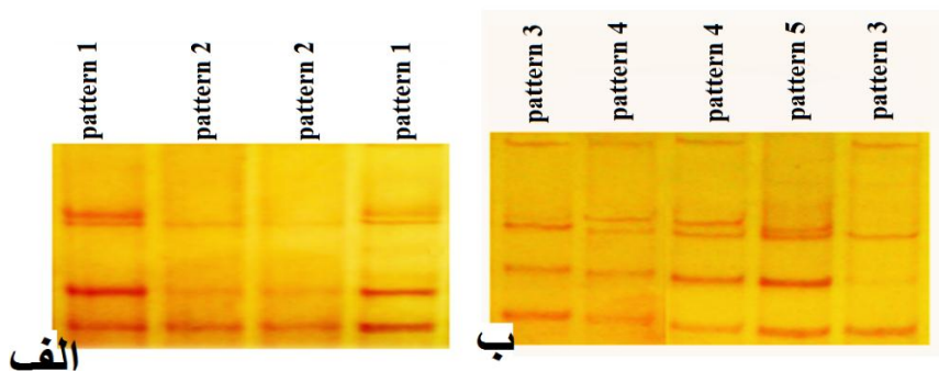
شکل ۲- تعداد ۵ الگوی باندی متفاوت به صورت الگوهای شماره ۱ تا ۵ (pattern 1-5) در نتایج SSCP از ناحیه افزونی ژن HSP70A1A (Oar_v4.0; Chr 20, NC_019477.2) در گوسفندان نژاد مهربان و رومانف. الف: دو الگوی متفاوت SSCP در قطعه ۲۴۷ جفت بازی که به pattern 1 و pattern 2 نامگذاری شده است. ب: سه الگوی متفاوت SSCP در قطعه ۲۹۸ جفت بازی که به pattern 3، pattern 4 و pattern 5 نامگذاری شده است.
