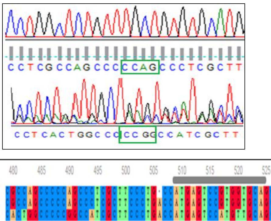
شکل ۳- جایجایی نوکلئوتیدی از نوع آدنین به گوانین در سایت برشی آنزیم MspI Figure 3. Nucleotide substitution from A to G in MspI palindrome
