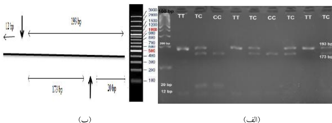
شکل ۳- (الف) طرح شماتیک محل تکثیر ژن PPARGC1α-T19C و هضم توسط آنزیم Bsur I را نشان می‌دهد (فلش‌ها جایگاه‌های شناسایی آنزیم می‌باشد). (ب) تعیین ژنوتیپ پلی مورفیسم T19C ژن PPARGC1α (به علت کوچک بودن بیش از حد قطعات ۲۰ و ۱۲ جفت بازی به سختی قابل تشخیص هستند).
