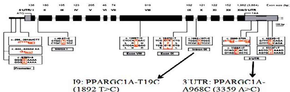
شکل ۱- نمای شماتیک ۱۱ چندشکلی ژن PPARGC1α (جایگاه‌های T19C و A968C با فلش مشخصند) Figure 1. Schematic picture of 11 polymorphisms of PPARGC1α (T19C and A968C is shown by arrow)
