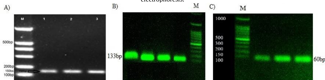
شکل ۲- الکتروفورز محصولات واکنش زنجیره ای پلیمراز. A: ژن بتاکتین B: اووئوئید C: اووآلبومین روی ژل آگارز ۲ درصد. M: مارکر مولکولی ۱۰۰ bp
