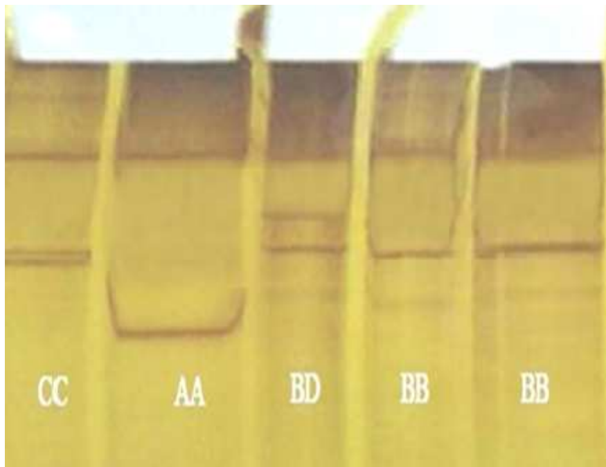
شکل ۲- الگوی باندی قطعات تکثیر شده جایگاه ۲ (اینترون ۱). در این جایگاه چهار الگوی باندی مشاهده شد که ژنوتیپ‌های AA و BB دو باند و ژنوتیپ‌های BD و CC دارای سه باند هستند.
