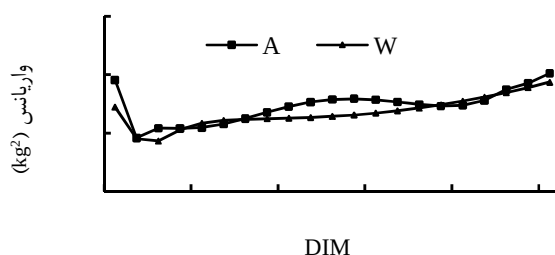
شکل ۳- واریانس ژنتیکی افزایشی به وسیله توابع ویلمینک (W) و علی- شیفر (A) در تابعی از روزهای شیردهی (DIM).
