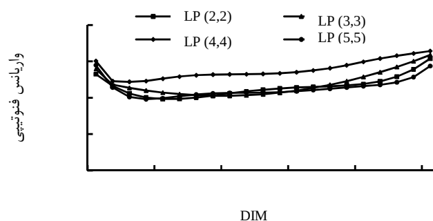
شکل ۶- واریانس فنوتیپی تولید شیر ( \text{kg}^2 ) به وسیله توابع چند جمله‌ای لژاندر (LP) در تابعی از روزهای شیردهی (DIM).
