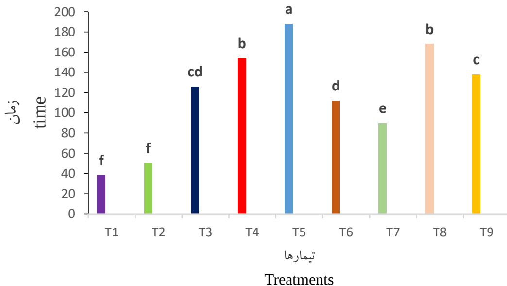
شکل ۲- اثر تفاله خرما بر پایداری هوازی سیلاژ یونجه
