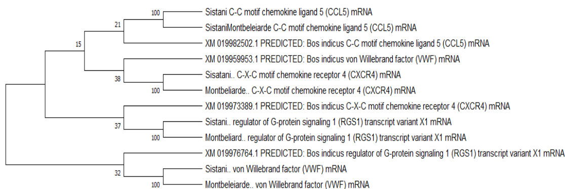
شکل ۲- درخت فیلوژنتیک توالی‌های نوکلئوتیدی چهار جایگاه ژنی مرتبط با صفات ایمنی در نژاد خالص سیستانی و آمیخته آن با مونت بیلارد Figure 2. Phylogenetic tree of nucleotide sequences of four loci gene related to immune traits in pure Sistani breed and its crosses with Montbeliarde
