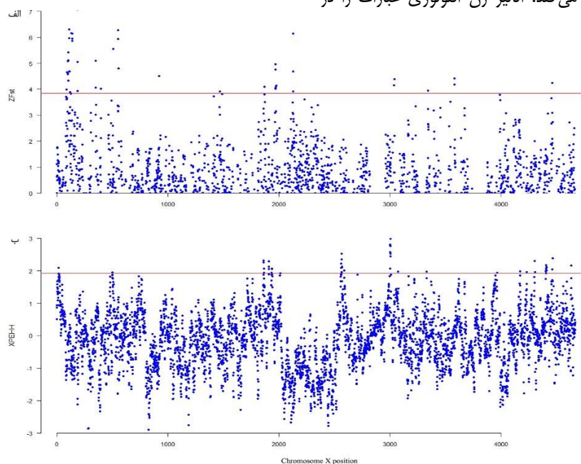
شکل ۱- نمودار منتهن پلات نواحی ژنومی شناسایی شده به عنوان نشانه‌های انتخاب در کروموزوم X در شتر تک‌کوهانه ایرانی با استفاده از روش ZFst (الف) و XP-EHH (ب)؛ خط قرمز نشان‌دهنده حد آستانه معنادار برای هر یک از روش‌ها است Figure 1. Manhattan plot of identified genomic regions as selection signatures on the X chromosome in Iranian dromedary camel using ZFst (a) and XP-EHH (b) methods; the red line indicates significant threshold for each methods
