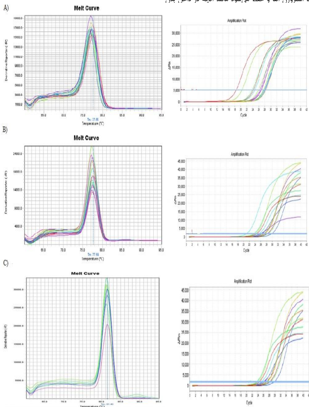
شکل ۳- منحنی تکثیر استاندارد (راست) و منحنی ذوب (چپ) مربوط به ژن‌های A: اووآلبومین B: اووموئید و C: بتا‌کتین حاصل از واکنش زنجیره‌ای پلیمرز در زمان واقعی برای مرغ تخمگذار
