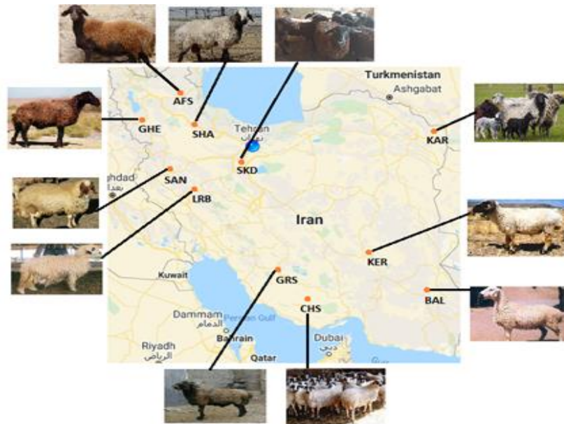
شکل ۱- شمای گرافیکی از توزیع جغرافیایی نژادهای گوسفند مورد مطالعه Figure 1. Graphic diagram of the geographical distribution of the studied sheep breeds: AFS=Afshari, KER=Kermani, GHE=Ghezel, GRS=Gray Shiraz, KAR=Karakul, BAL=Baluchi, LRB=Lori Bakhtiari, SAN=Sanjabi, SHA=Shal, SKD=Siah Kabud, CHS= Chios
