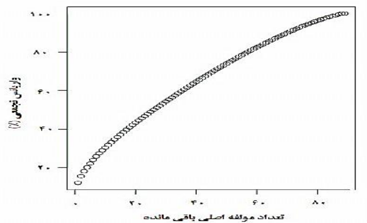
شکل ۲- میزان واریانس تجمعی توجیه شده بر حسب تعداد مؤلفه‌های اصلی باقی مانده Figure 2. The cumulative variance explained by residual principle components remained in model
