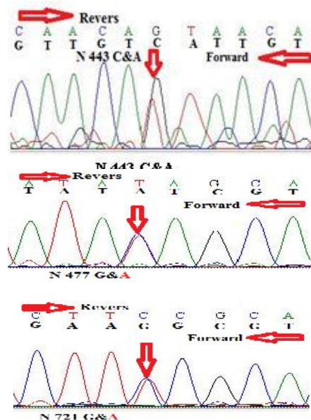
شکل ۳- کروماتوگرام حاصل از نتایج توالی‌یابی برای SNPهای هتروزیگوت شناسایی شده جایگاه نیمه اول اگزون ۲ ژن GDF9 Figure 3. Achieved chromatogram from sequencing for detected heterozygous SNPs in the first half of exon 2 of GDF9 gene
