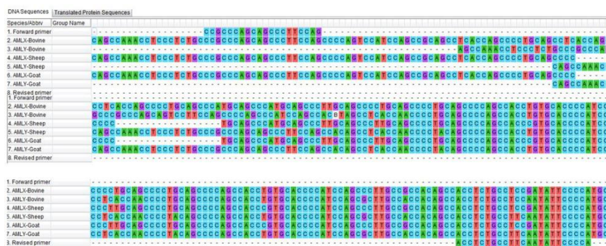
شکل ۲- توالی نوکلئوتیدی ژن آمیلوژنین (ژن کاندیدا) در گاو، گوسفند و بز (آغازگر برای قسمتی از ژن که داخل کادر سیاه است طراحی می شود) Figure 2. Sequence of amelogenin gene in bovine and ovine and caprine species
