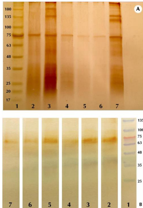
شکل ۲- (A) SDS-PAGE [۱- مارکر؛ ۲- سویه استاندارد (RTCC 2375)؛ ۳ تا ۷ نمونه سرم‌ها] و (B) تست وسترن بلات برای سرم‌ها [۱- مارکر؛ ۲- کنترل مثبت سویه استاندارد (RTCC 2375)؛ ۳ تا ۷ سرم‌ها] Figure 2. (A) SDS-PAGE [1- marker; 2- Standard strain (RTCC 2375); 3 to 7 samples of serums] and (B) Western blot test for serums [1- marker; 2- Standard strain positive control (RTCC 2375); 3 to 7 serum]
