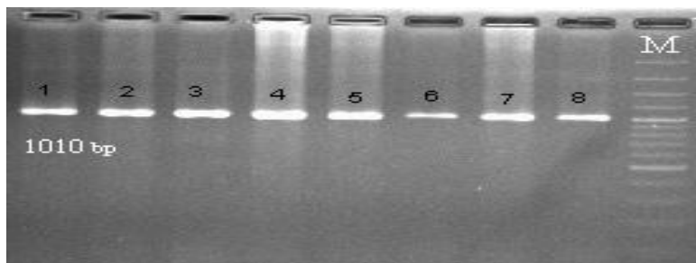
شکل ۳- الکتروفورز محصولات حاصل از هضم توسط آنزیم BstEII در جایگاه ژنی PEPCK-C (3). چاهک ۱-۳ مرغ تخم‌گذار، ۴-۶ مرغ گوشتی و ۷-۹ مرغ بومی. ژنوتیپ BB در همه نمونه‌های مورد بررسی مشاهده شد، M خط کش مولکولی ۱۰۰ جفت بازی. Figure 3. Electrophoresis of digestion products by BstEII enzyme in PEPCK-C (3) locus. Lane 1-3 layer, 4-6 broiler and 7-8 native fowls. BB genotype observed in all samples. M is the 100bp molecular ruler
