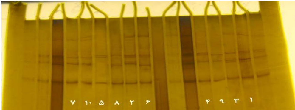
شکل ۳- پلی مورفیسیم حاصل از تکنیک SSCP در ژن لپتین در گوسفند آمیخته لری بختیاری - افشاری با ۱۰ الگوی متفاوت Figure 3. SSCP polymorphism of Lori Bakhtiari- Afshari Hybrid sheep in leptin gene with ten different patterns (genotype)
