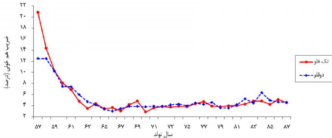
شکل ۴- روند تغییرات میانگین ضریب هم خونی (درصد) بره‌های تک و دوقلو در بین حیوانات هم‌خون
